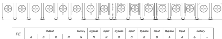
(б) Силовые клеммы ИБП мощностью 10-60 кВА с отсеком для встроенных АКБ
