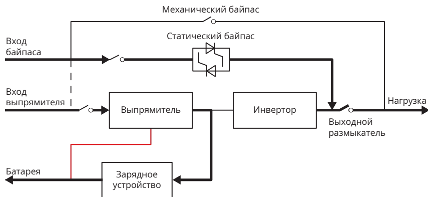
Рисунок 2.6. Функциональная схема ИБП при работе в режиме байпаса
