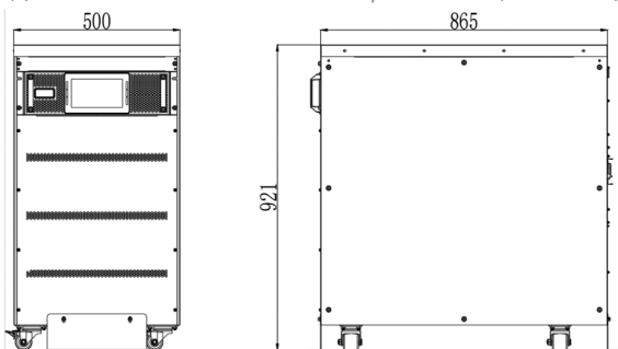
(г) 10; 15; 20; 30 кВА с отсеком для встроенных АКБ (ед. изм.: мм)
