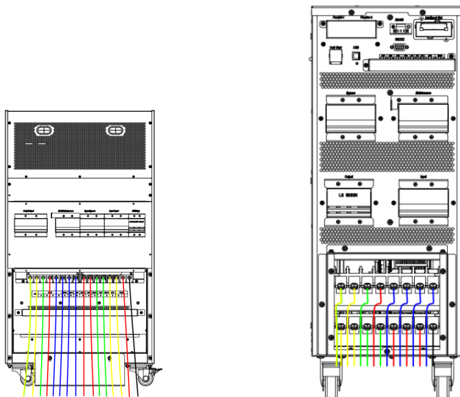
Рисунок 3.6. Кабельный ввод
