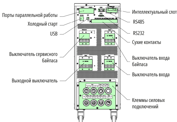
(а) 10-40 кВА без отсека для встроенных АКБ
