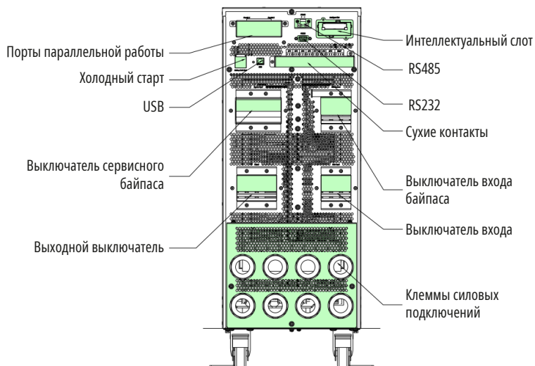
(д) ИБП мощностью 40/60 кВА без отсека для встроенных АКБ, вид сзади
