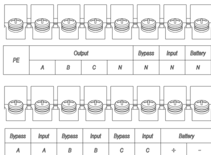
(а) Силовые клеммы ИБП мощностью 10-40 кВА без отсека для встроенных АКБ
