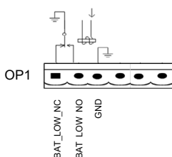
Рисунок 3.13. Схема интерфейса выходного релейного контакта предупреждения о низком напряжении АКБ
