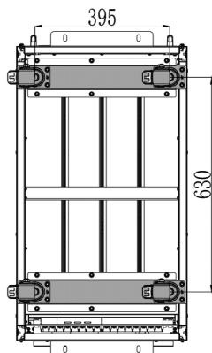
(б) ИБП 10 – 80 кВА с отсеком для встроенных АКБ (вид снизу, ед. изм.: мм)
