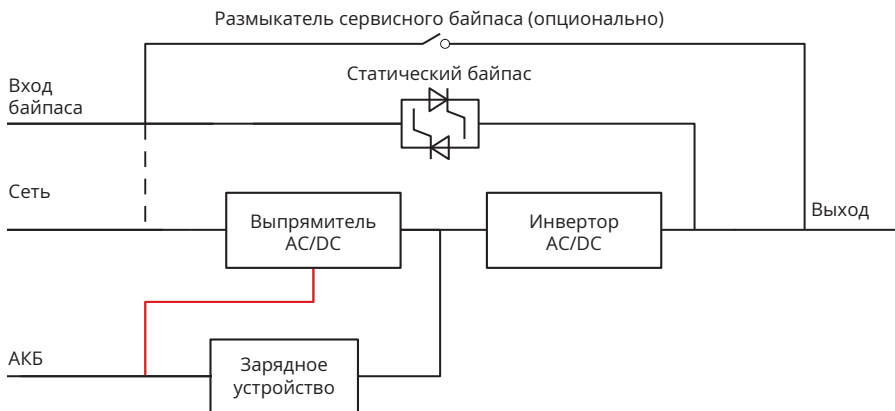
Рисунок 2.3. Структура ИБП
