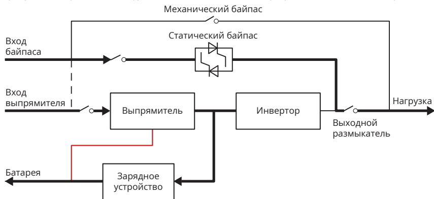
Рисунок 2.8. Функциональная схема ИБП при работе в экономичном режиме
