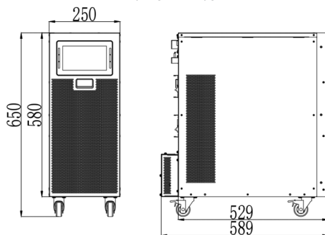
(а) 10 / 15 / 20 кВА без отсека для встроенных АКБ (ед. изм.: мм)
