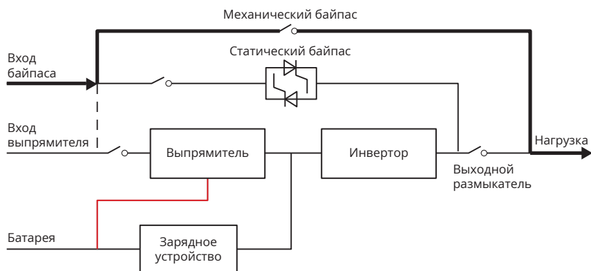
Рисунок 2.7. Функциональная схема ИБП при работе в режиме сервисного байпаса
