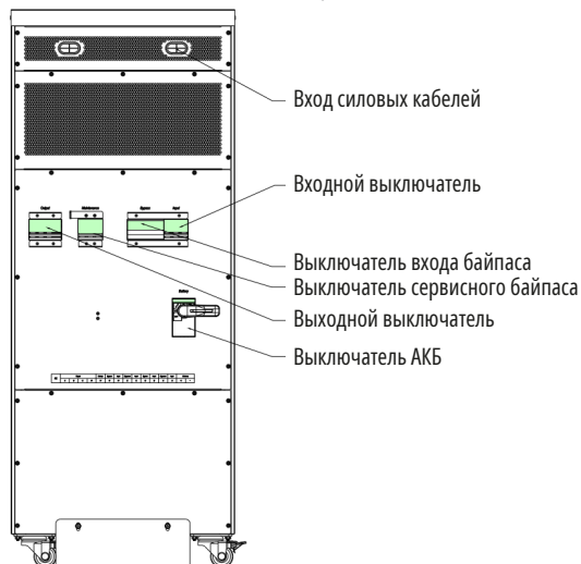
(ж) ИБП мощностью 60-80 кВА с отсеком для встроенных АКБ, вид сзади
