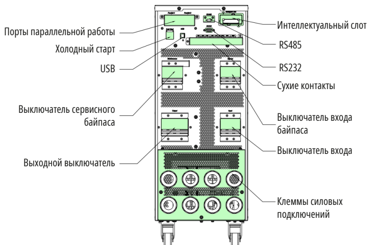
(г) ИБП мощностью 10-30 кВА без отсека для встроенных АКБ, вид сзади
