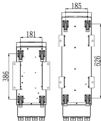
(а) ИБП 10-30 кВА и 40 кВА без отсека для встроенных АКБ (вид снизу, ед. изм.: мм)
