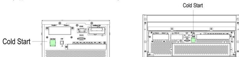
Рисунок 5.1. Расположение кнопки холодного запуска АКБ
