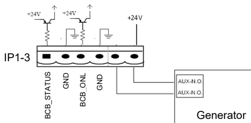
Рисунок 3.11. Схема входного порта для входа генератора
