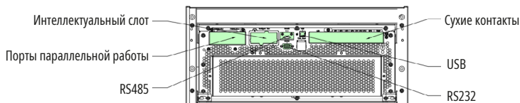
(в) 40 кВА с отсеком для встроенных АКБ
