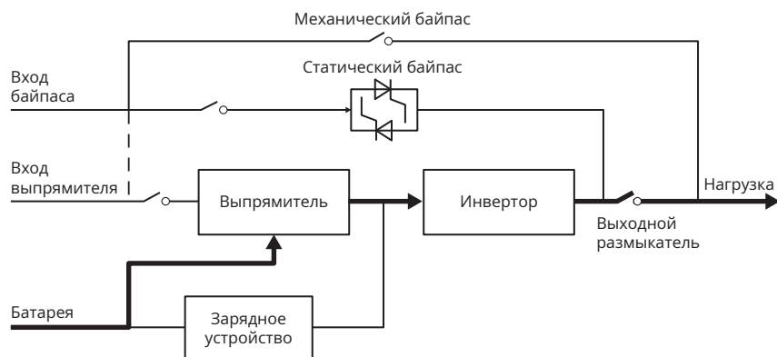
Рисунок 2.5. Функциональная схема ИБП при работе от АКБ
