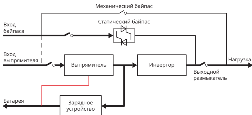
Рисунок 2.4. Функциональная схема нормального режима работы
