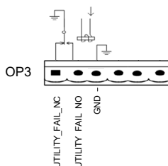
Рисунок 3.15. Схема интерфейса выходного релейного контакта предупреждения отказа сети
