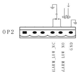
Рисунок 3.14. Схема интерфейса выходного релейного контакта общей тревоги
