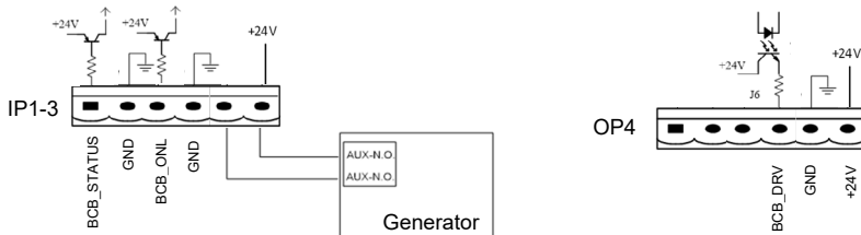
Рисунок 3.12. Порт АВ АКБ
