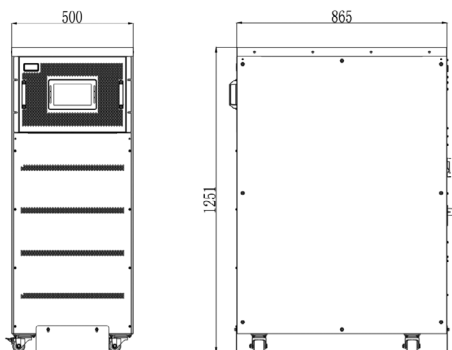
(е) 60 / 80 кВА с отсеком для встроенных АКБ (ед. изм.: мм)
