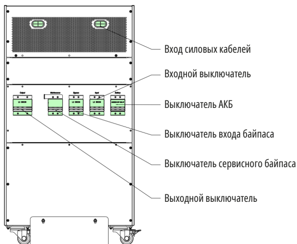
(е) ИБП мощностью 10-40 кВА с отсеком для встроенных АКБ, вид сзади
