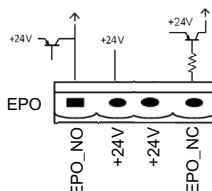
Рисунок 3.9. Схема входного порта для дистанционной подачи команды EPO
