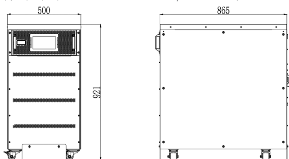
(д) 40 кВА с отсеком для встроенных АКБ (ед. изм.: мм)
