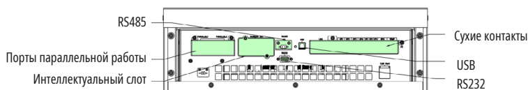
Рисунок 3.8. Коммуникационные интерфейсы и «сухие» контакты
