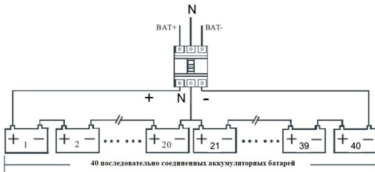
Рисунок 3.5. Схема подключения АКБ
