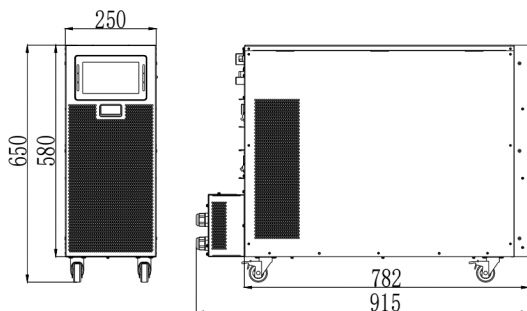
(в) 40 / 60 / 80 кВА без отсека для встроенных АКБ (ед. изм.: мм)
