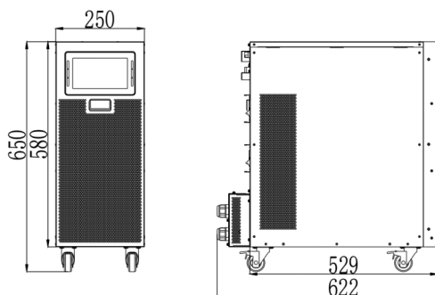
(б) 30 кВА без отсека для встроенных АКБ (ед. изм.: мм)
