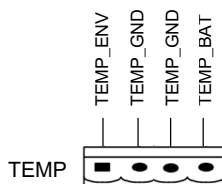
Рисунок 3.10. Порты TEMP 1-4 для определения температуры
