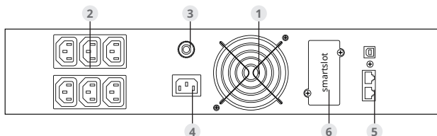
Рис. 2.3.2. Задняя панель ИБП в стойку (ЮНИОР ПРО RT) 1000 ВА 2U
