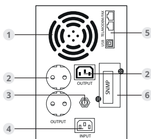
Рис. 2.3.1. Задняя панель напольного ИБП 1000-2000 ВА
