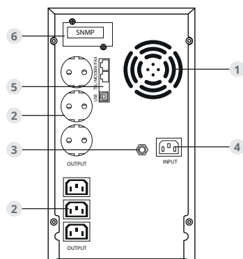
Рис. 2.3.1. Задняя панель напольного ИБП 3000 ВА
