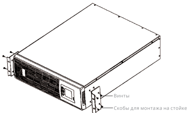
Рис. 3.2.4.3. Установка креплений для монтажа в стойку
