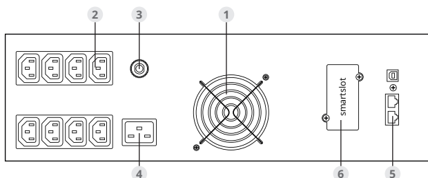
Рис. 2.3.2. Задняя панель ИБП в стойку (ЮНИОР ПРО RT) 2000 - 3000 ВА 3U
